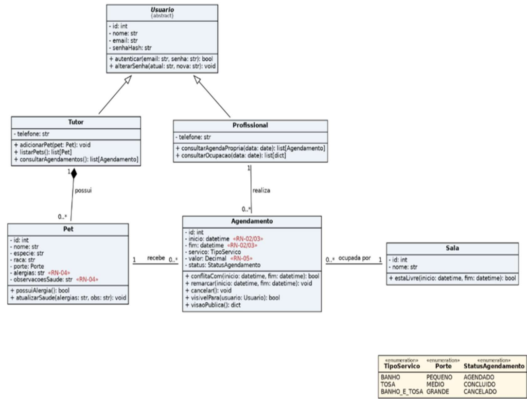
Figura 2 — Diagrama de classes (atributos em vermelho refletem regras de negócio)
